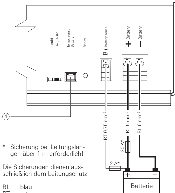
Bild 4: Anschlussplan
