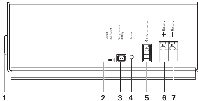
Bild 1: Anschlüsse
