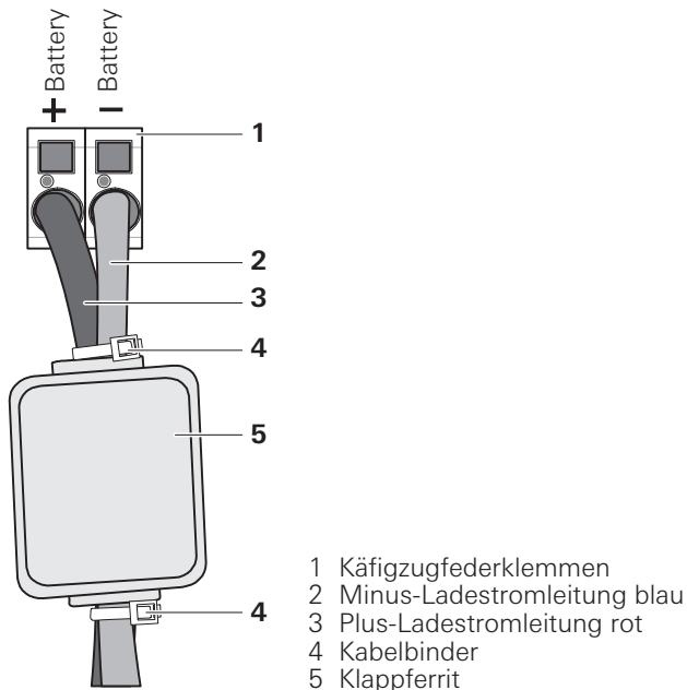
Bild 3: Klappferrit
