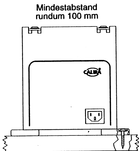
Bild 3: Montage
