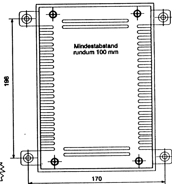
Bild 4: Montage
