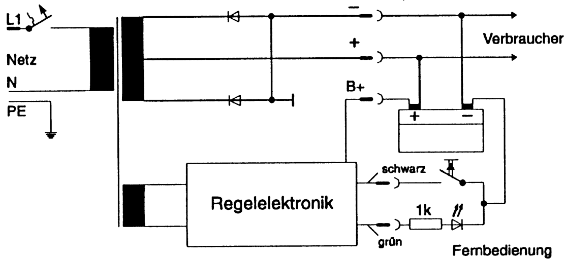
Bild 1: Blockschaltbild
