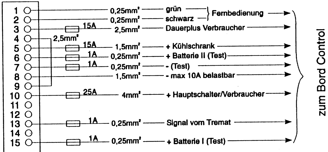
Bild 5: Anschlußplan 15 poliger Steckverbinder
