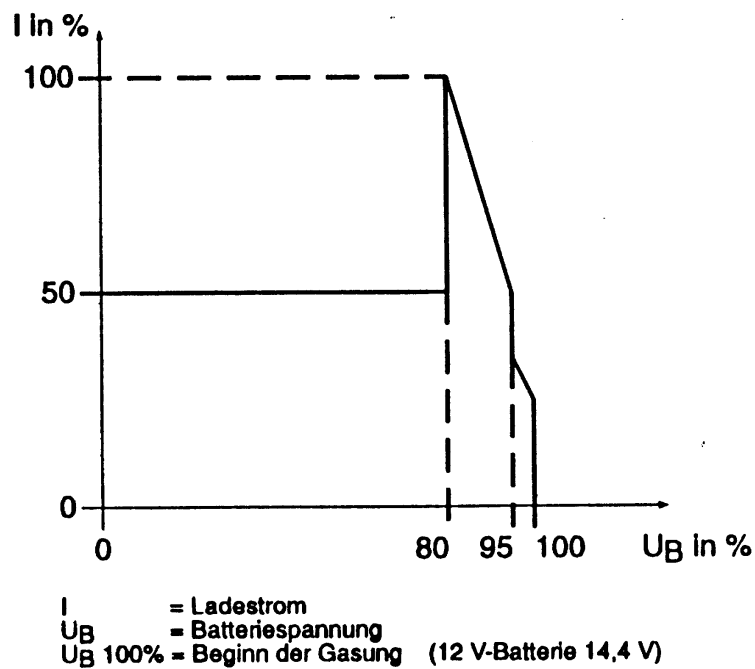
Bild 2: Ladekennlinie (prinzipieller Verlauf)
