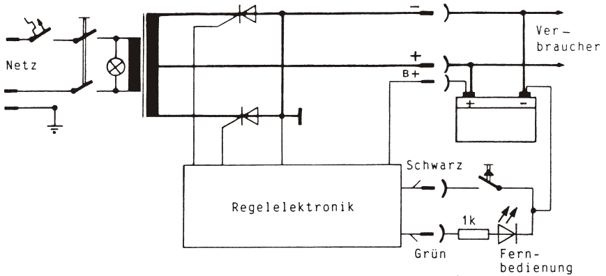
Bild 1: Blockschaltbild
