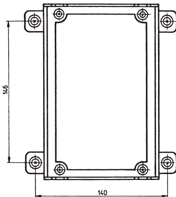
Bild 3: Befestigungsschema
