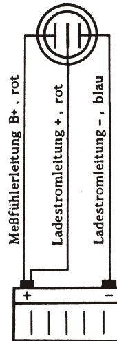
Bild 4: Anschlußschema
