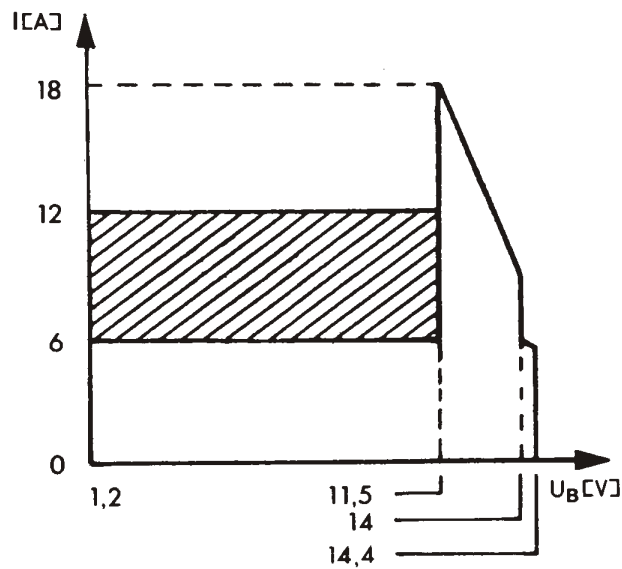
Bild 2: Ladekennlinie (prinzipieller Verlauf)
