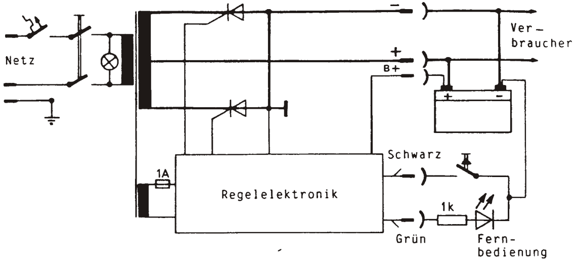
Bild 1: Blockschaltbild
