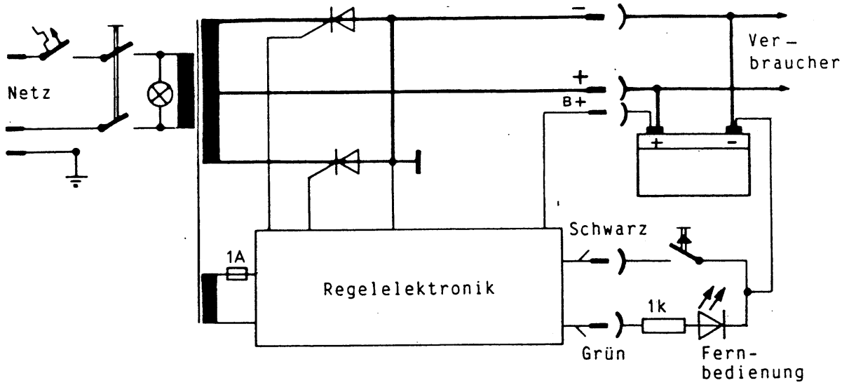
Bild 1: Blockschaltbild
