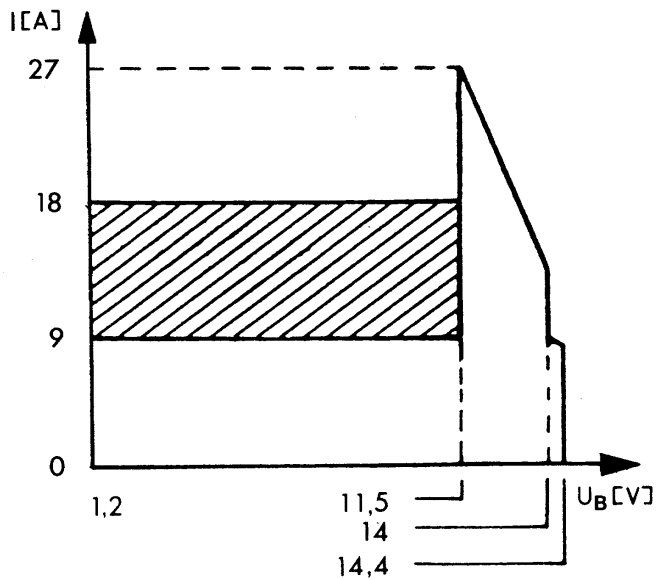
Bild 2: Ladekennlinie (prinzipieller Verlauf)
