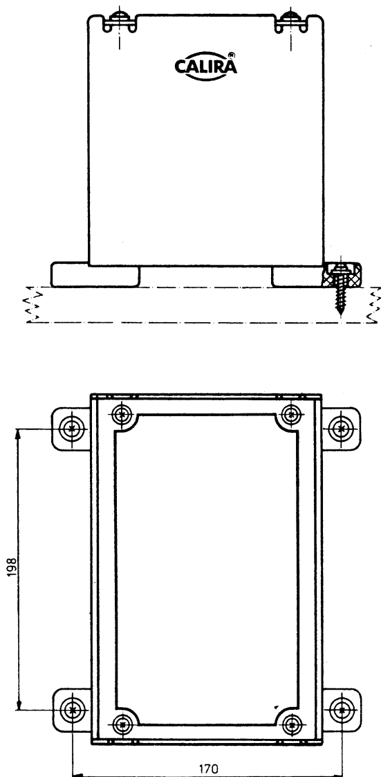
Bild 3: Befestigungsschema
